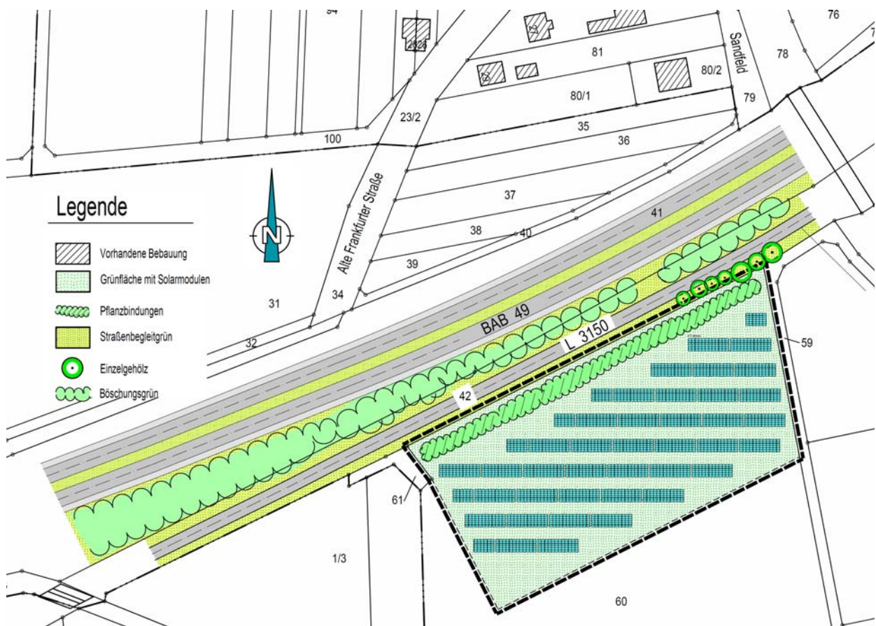
Entwicklungsskizze
