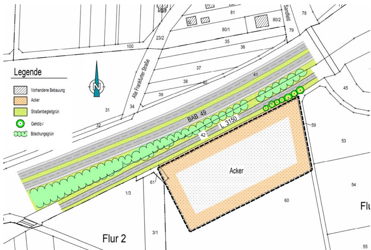
Bestandsplan ohne Maßstab
